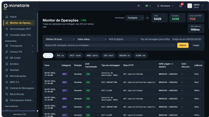
Monitor: tabela sem UNKNOWN, rotulada por funcao
